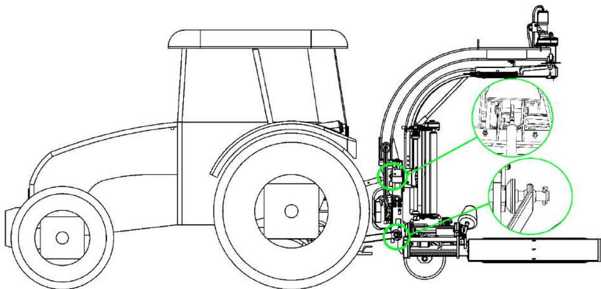
рисунок 7. Точки соединения трактора с обмотчиком
