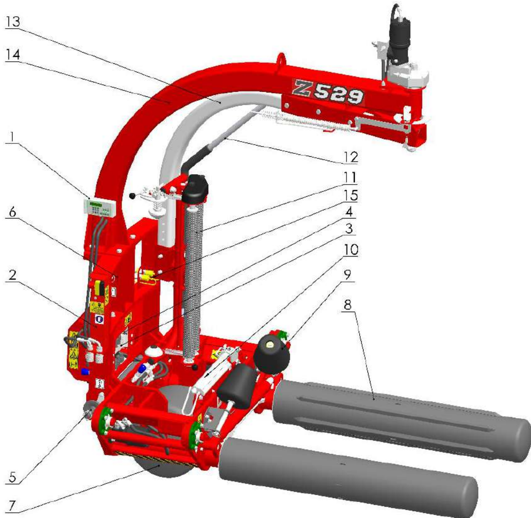
рисунок 3. Устройство обмотчика
