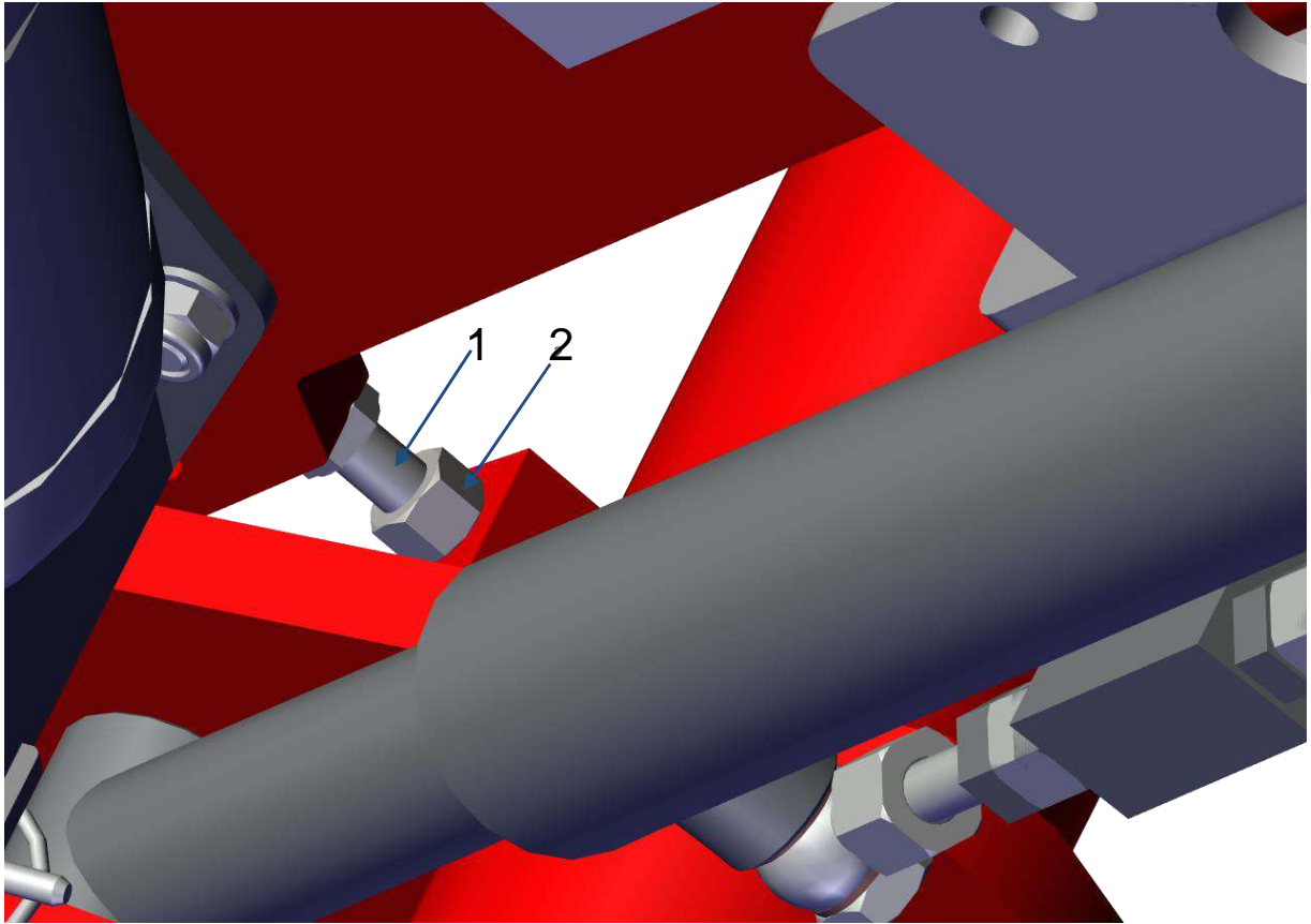
рисунок 36. Ограничение складывание плеч
