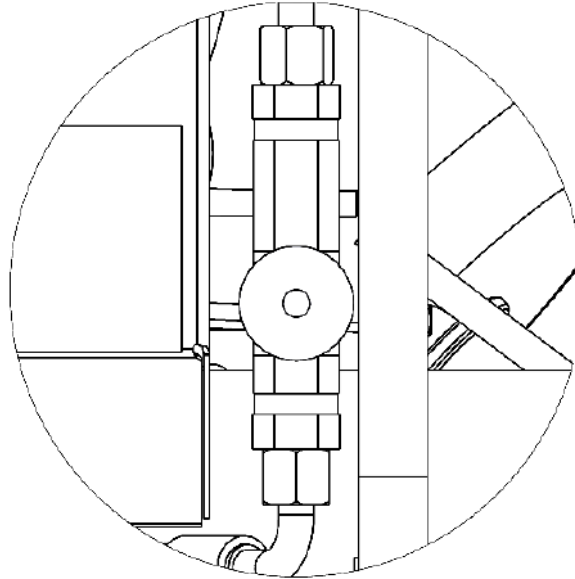
рисунок 27. Обратно-дроссельный клапан нижних плеч и механизма установки рулонов
