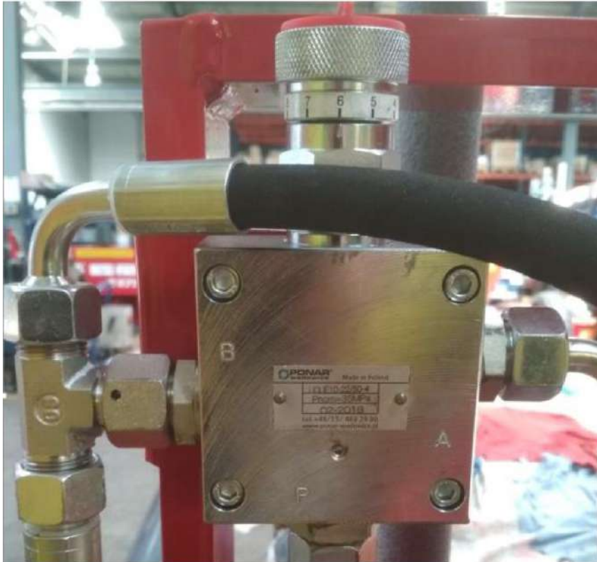
рисунок 30. Регулятор расхода
