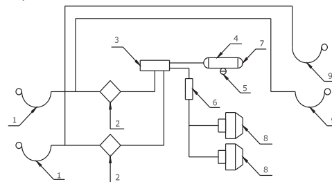
Рис. 3 Схема пневматической двухпроводной тормозной системы. 1 – пневматический соединительный элемент первого прицепа, 2 – воздушный фильтр, 3 – управляющий клапан, 4 – воздушный бак, 5 – водоотводящий клапан, 6 – ручной регулятор силы торможения, 7 – контрольное соединение, 8 – мембранный пневмоцилиндр, 9 – пневматический соединительный элемент второго прицепа.
